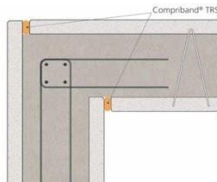
Croquis : Joint béton / liaison d'angle
