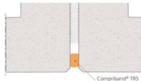
Croquis : Joint entre éléments de béton branché
