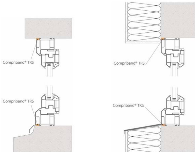
Croquis : Pose en tunnel
