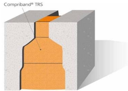
Croquis : Etanchéité avec plusieurs d'utilisation plages d'utilisation
