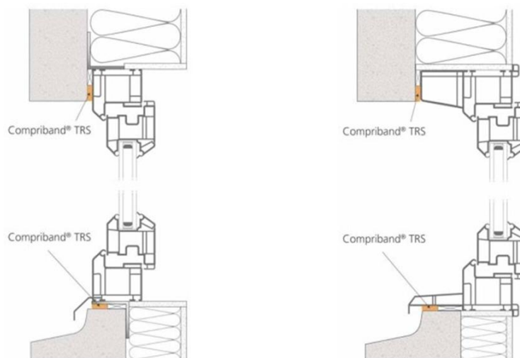
Croquis : Pose en applique intérieure avec appui décalé
