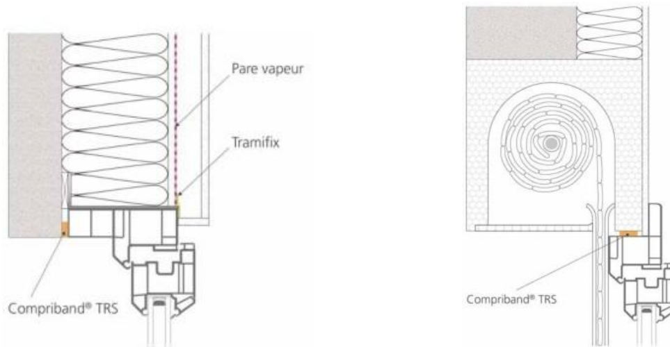
Croquis : Exemples d'étanchéité sous linteau
