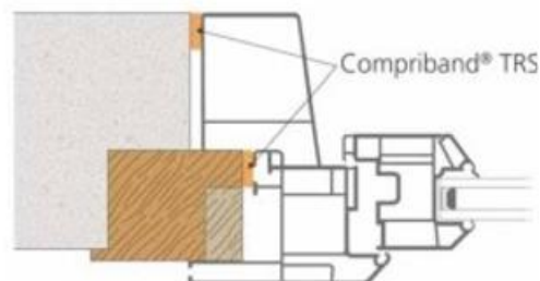
Croquis : Mise en œuvre en rénovation
