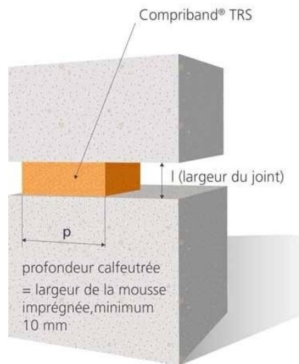
Croquis : Coupe transversale du joint
