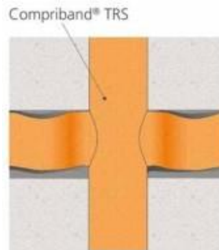
Croquis : Raccord en croix
