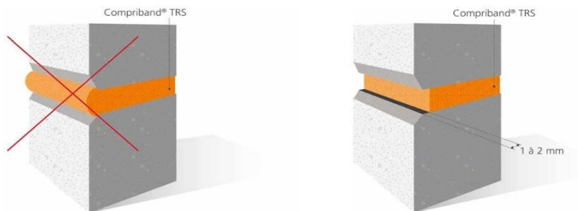
Croquis : Positionnement dans le joint
