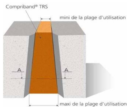
Croquis : Etanchéité avec plage
