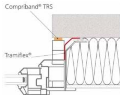
Croquis : Exemples d'étanchéité entre tableau et menuiserie
