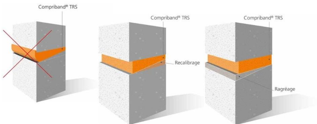
Croquis : Surface de contact
