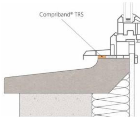
Croquis : Exemple d'étanchéité sous pièce d'appui
