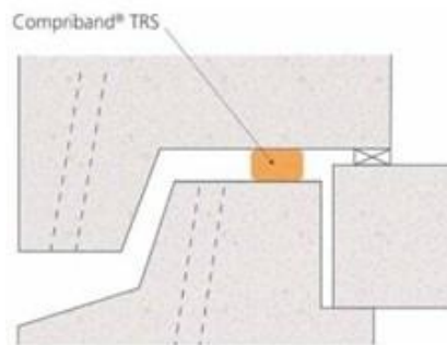
Croquis : Sous-élément préfabriqués lourds
