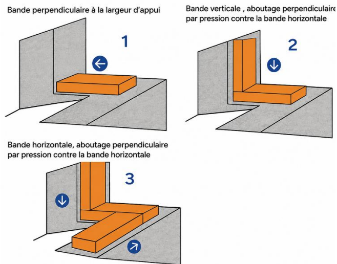
Croquis : Raccords en trois bandes sur rejingot (pose applique)
