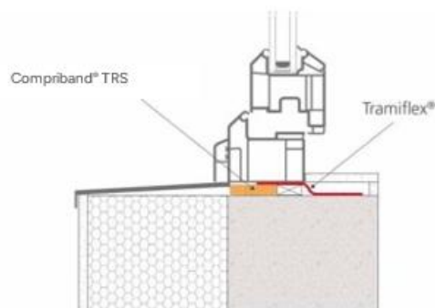
Croquis : Exemple d'étanchéité sous pièce d'appui
