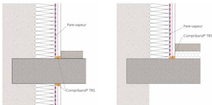
Croquis : Etanchéité du doublage sur mur en maçonnerie
