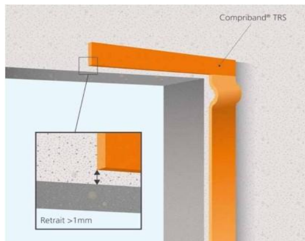
Croquis : Raccord d'angle de deux extrémités continues (pose applique)
