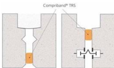
Croquis : Sous-élément préfabriqués lourds
