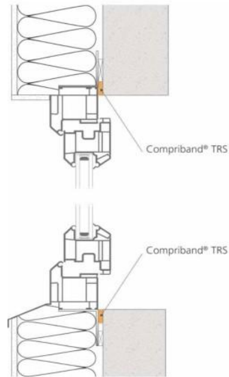
Croquis : Pose en applique extérieure
