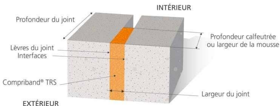
Croquis : Terminologie relative aux joints
